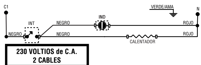
DIAGRAMA DE CONEXIONES WX1A
