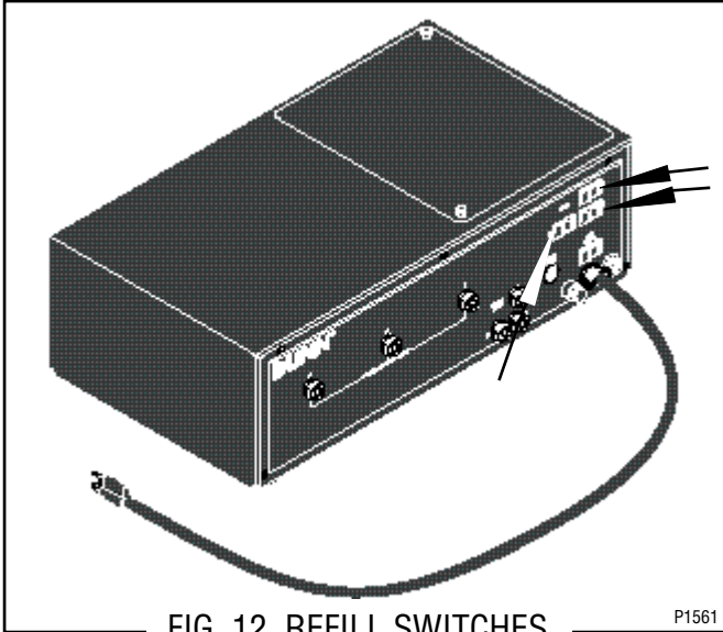
FIG. 12 REFILL SWITCHES
